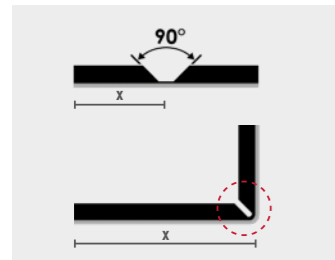
1. FRÄSNUT 90°
